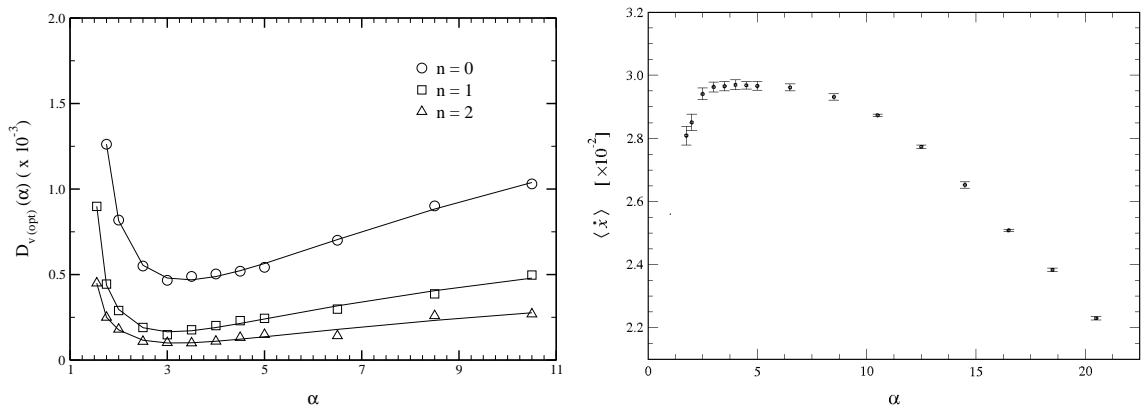
Figura 5.1: Condições de otimização para dois sistemas distintos. À esquerda, curvas de otimização na dinâmica neural. À direita, otimização do transporte de partículas num motor browniano unidimensional. As duas condições de otimização foram obtidas para um comportamento estocástico fortemente não-gaussiano.
